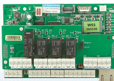
WS4-2D-E electrónica del WS4-2D
